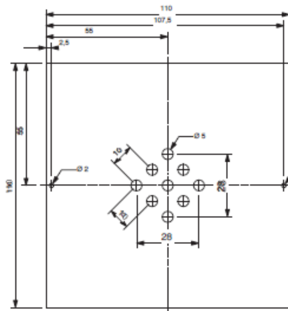
Deckplatte (1b)
