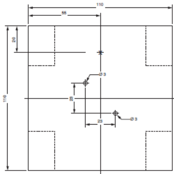
Grundplatte (1a)
